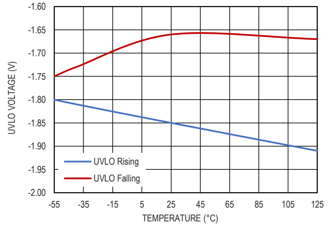
图 16. UVLO 阈值和结温的关系
