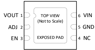
图 3. 2mm x 2mm DFN6 引脚配置(顶视图)
