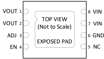
图 2. 3mm x 3mm DF8N 引脚配置(顶视图)
