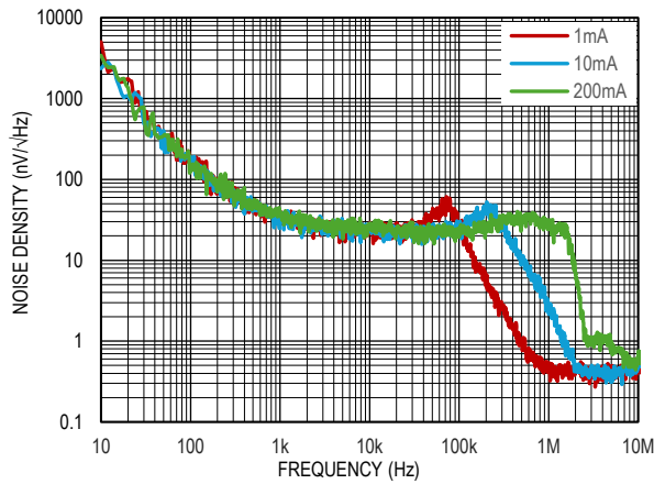
图 13. 噪声谱密度
