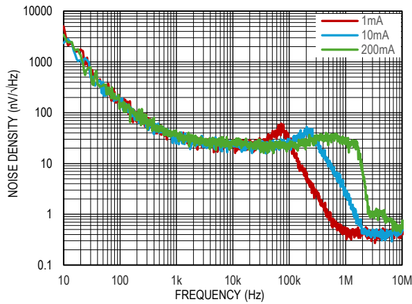
图 10. 噪声谱密度
