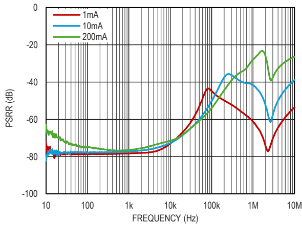
图 12. PSRR 和负载电流的关系
