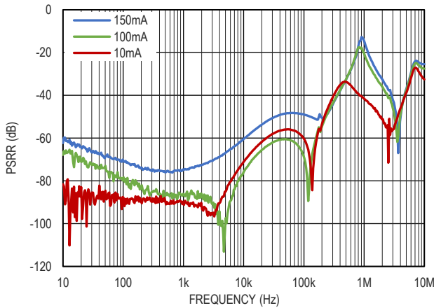
图 18. 电源电压纹波抑制比与负载的关系, V_{OUT}=3.3V
