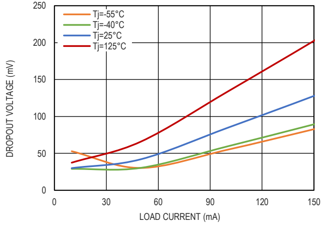
图 4. 3.3V 压差电压和负载电流的关系
