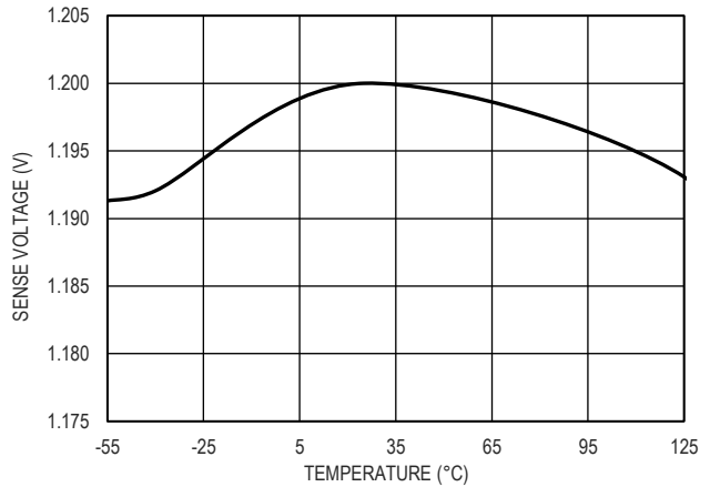
图 11. 1.2V SENSE 引脚电压精度
