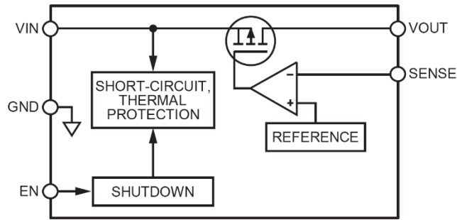
图 22. 内部框图
