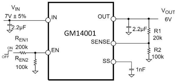
图 26. EN 引脚的典型分压器
