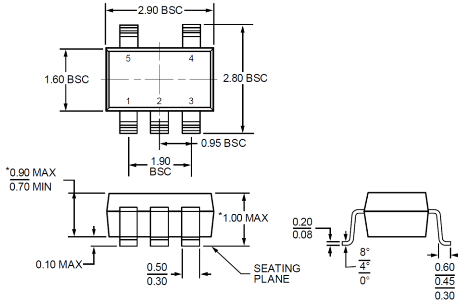
图 28.5 引脚超薄 SOT
