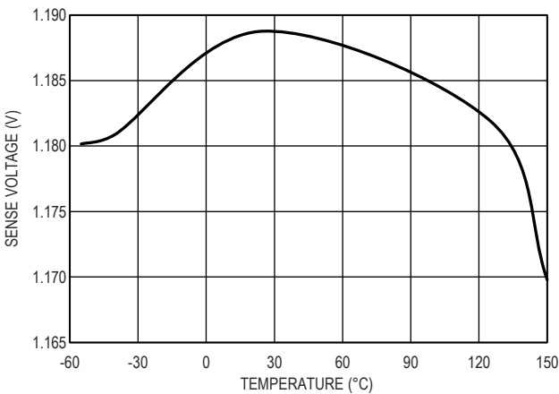
图 12. 1.2V SENSE 引脚电压精度
