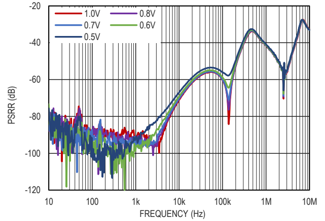
图 17. 电源电压纹波抑制比与压差的关系, V_{OUT}=5.0V
