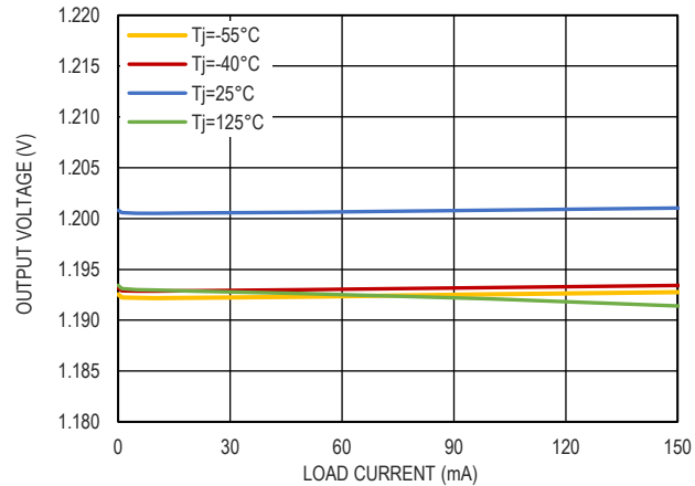
图 8. 1.2V 输出电压和负载电流的关系
