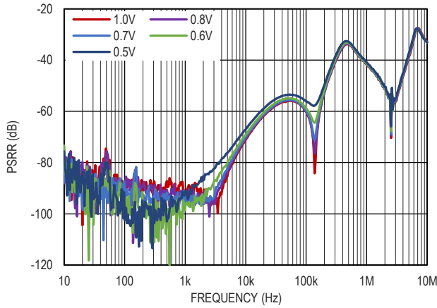
图 16. 电源电压纹波抑制比与压差的关系, V_{OUT}=3.3V
