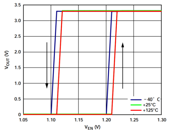
图 25. 对 EN 引脚工作方式的典型 V_{OUT} 响应
