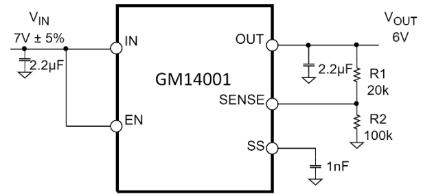
图 23. 典型可调输出电压应用原理图
