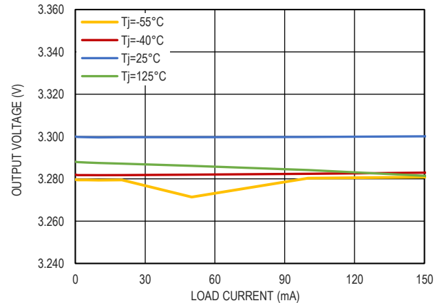
图 9. 3.3V 输出电压和负载电流的关系
