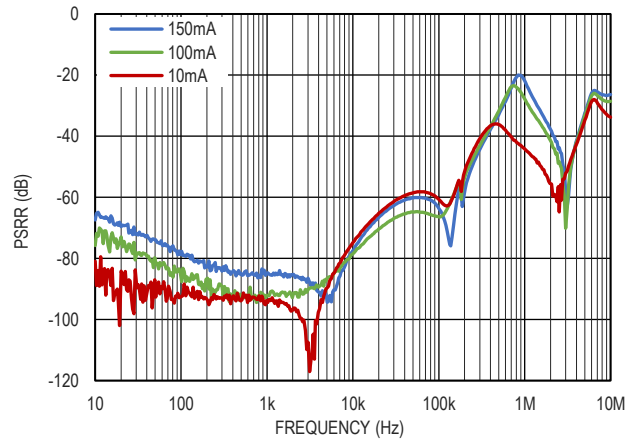
图 19. 电源电压纹波抑制比与负载的关系, V_{OUT}=5.0V
