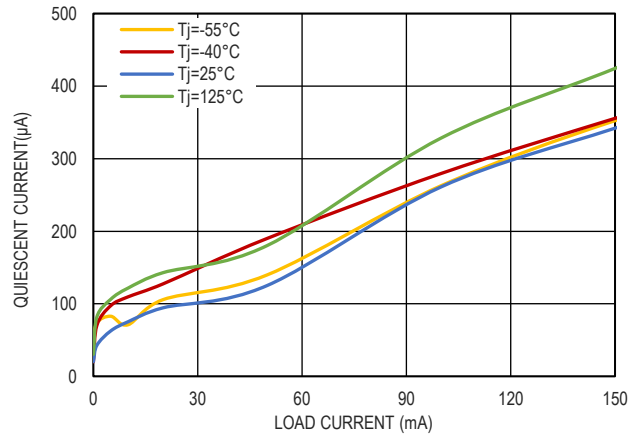
图 6. 静态电流和负载电流的关系, V_{IN} = 4.3V
