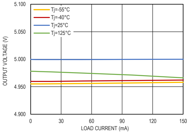
图 10. 5.0V 输出电压和负载电流的关系
