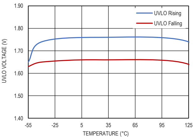
图 14. UVLO 阈值和温度的关系
