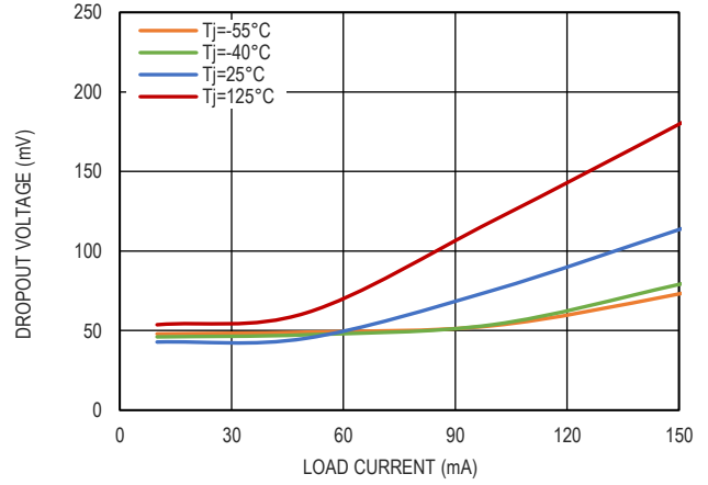
图 5. 5.0V 压差电压和负载电流的关系
