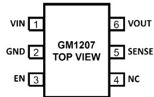
图 5.6 引脚 SOT-23 引脚配置
