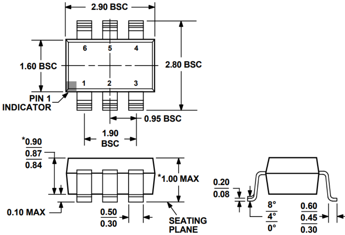
图 33.6 引脚 SOT-23
