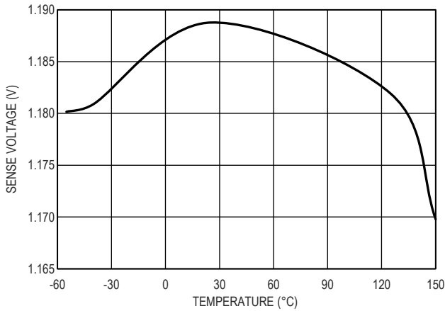
图 14. 1.188V SENSE 引脚电压精度
