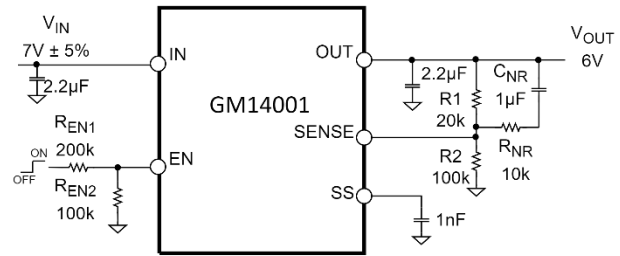
图 29. 噪声优化
