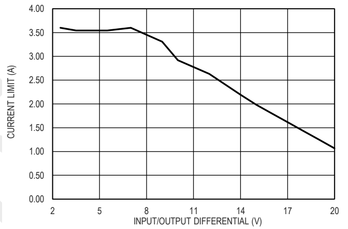
图 13. 输出限流值和输入输出压差的关系
