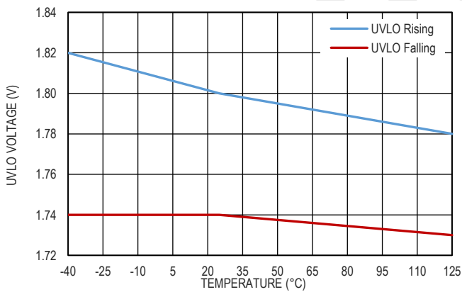
图 14. UVLO 阈值
