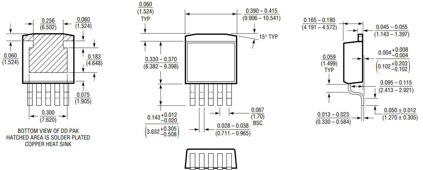
图 21.5 引脚 TO-263
