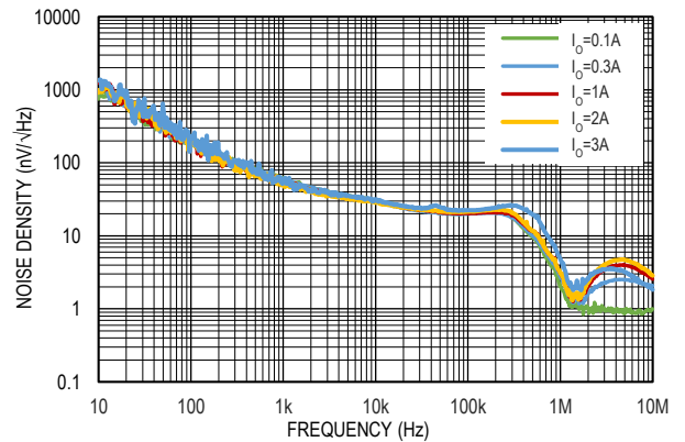
图 15. 输出噪声谱密度, V_{IN}=5V , V_{OUT}=3.3V
