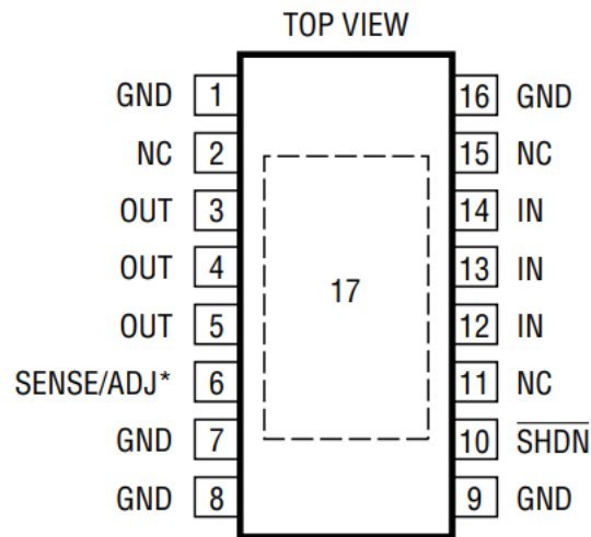
16 引脚 TSSOP 裸露焊盘必须焊接到 PCB 上
