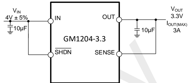
图 1 典型应用
