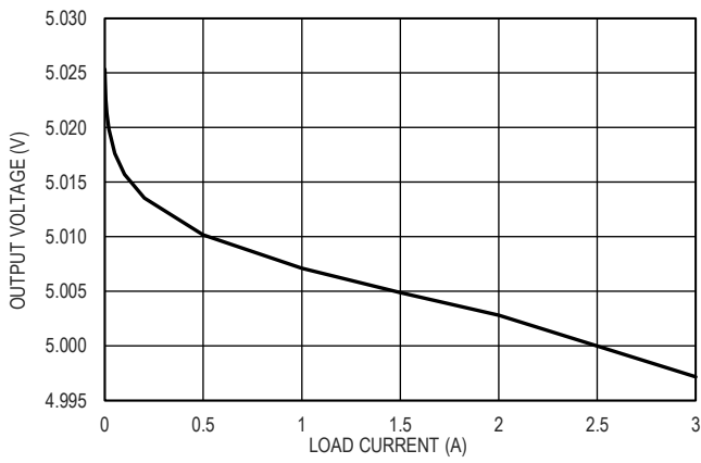
图 10. 5.0V 输出电压和负载电流的关系
