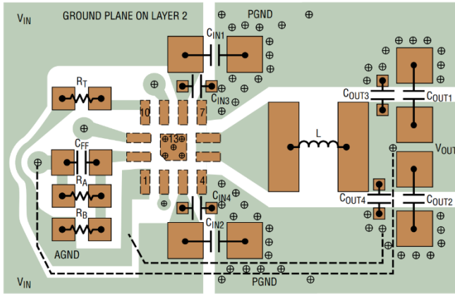
图 6. 推荐的 PCB 布局
