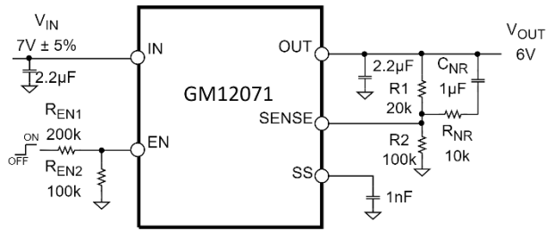
图 28. 噪声优化
