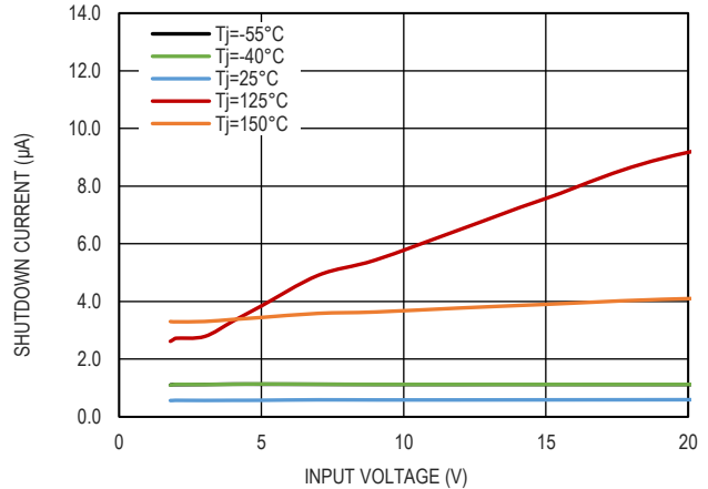
图 8. 关机电流和输入电压的关系
