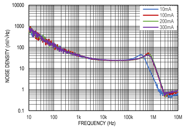
图 16. 输出噪声谱密度, V_{\text{IN}}=5\text{V} , V_{\text{OUT}}=3.3\text{V}
