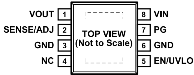
图 4.8 引脚 SOP-8 的引脚配置
