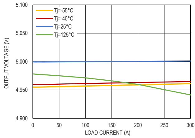
图 11. 5.0V 输出电压和负载电流的关系
