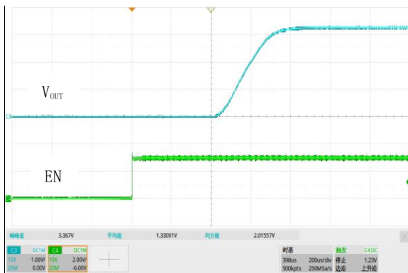
图 21. 软启动, V_{IN}=4.3V , V_{OUT}=3.3V , I_{OUT}=500mA
