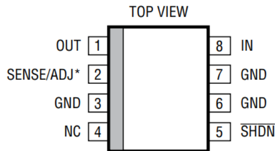
8 引脚 SOP 图 2 引脚配置
